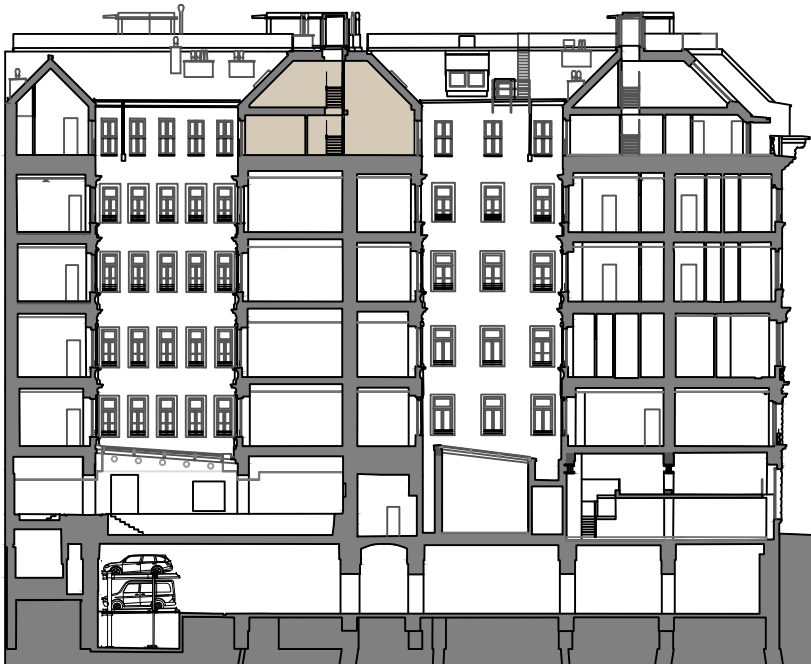
SCHNITT E-E
