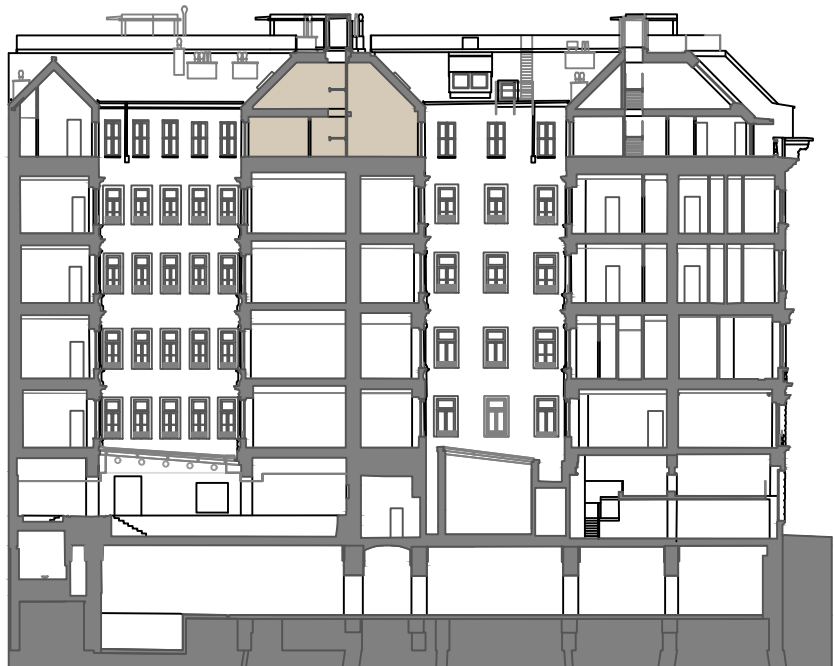
SCHNITT E-E
